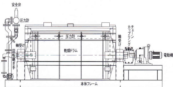
(側面図)
