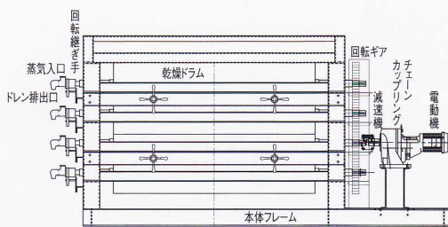
(側面図)
